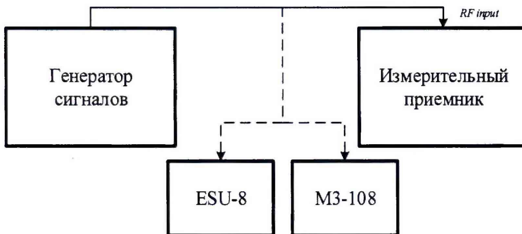
Рисунок 2. Схема подключения для определения допустимой абсолютной погрешности измерений уровня сигнала
