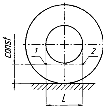
Рисунок 3 – Схема установки измерительных наконечников
