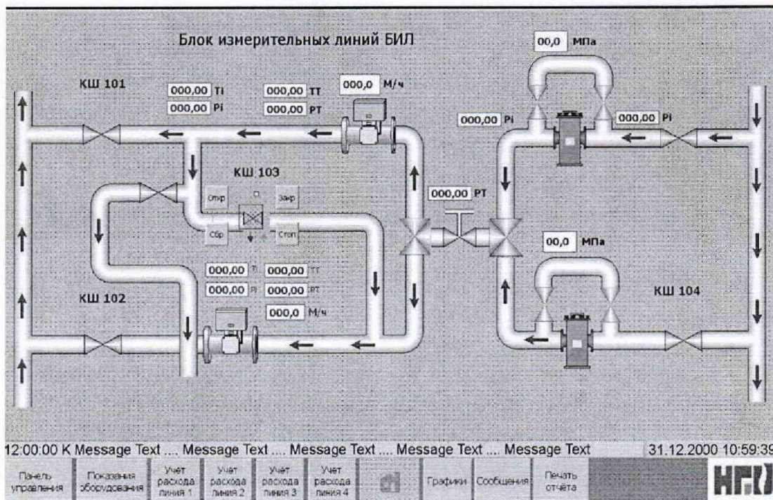
Рисунок 1 – Меню НМИ панели контроллера для отображения идентификационных данных
