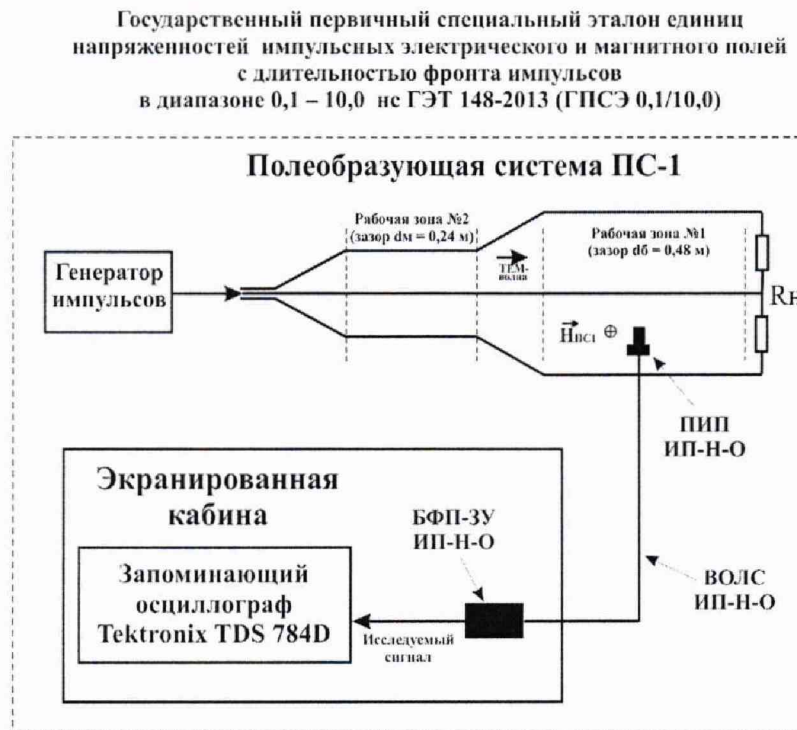
Рисунок 1 – Схема исследований при определении характеристик ИП-Н-О с использованием ГЭТ 148-2013 для воспроизведения единиц НИЭМП в диапазоне от 0,1 до 10,0 нс
