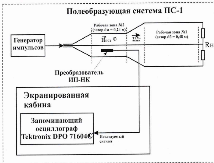
Рисунок 1 – Схема исследований при определении характеристик ИП-НК с использованием ГЭТ 148-2013 для воспроизведения единиц НИЭМП в диапазоне от 0,1 до 10,0 нс
