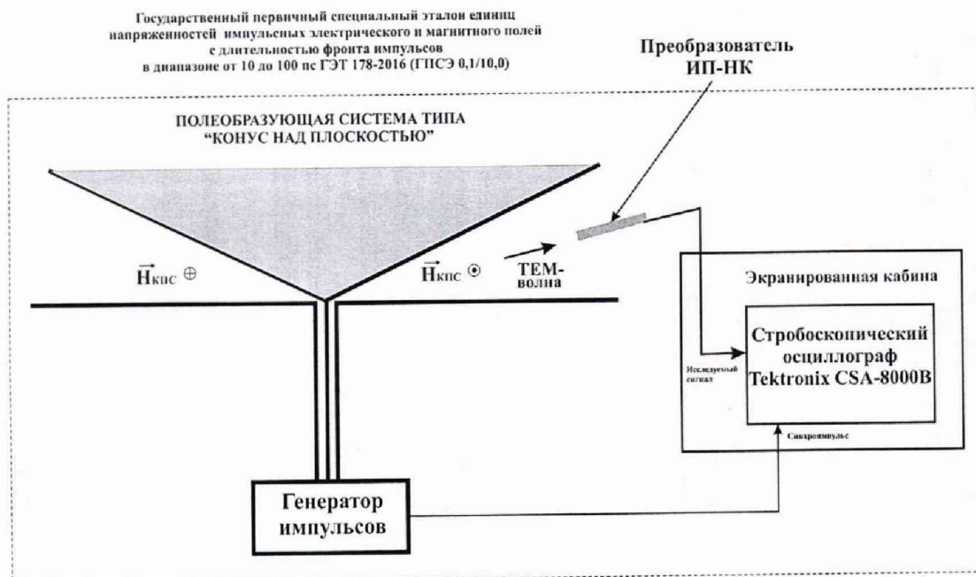
Рисунок 3 – Схема исследований при определении характеристик ИП-НК с использованием ГЭТ 178-2016 для воспроизведения единиц НИЭМП в диапазоне от 10 до 100 пс
