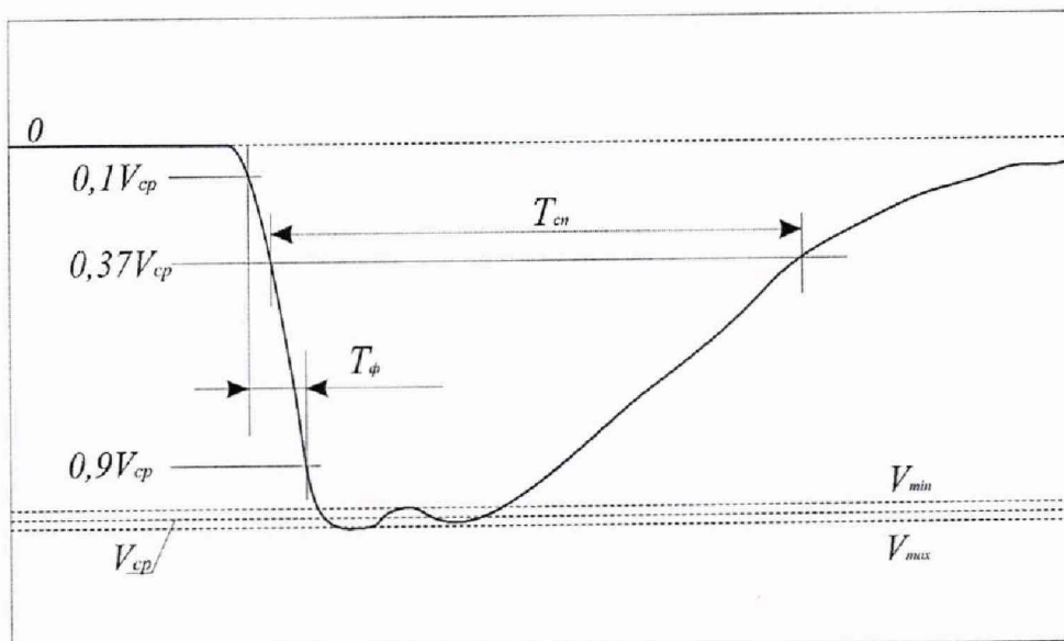
Рисунок 2 – Эюра напряжения на выходе преобразователя при определении метрологических характеристик
