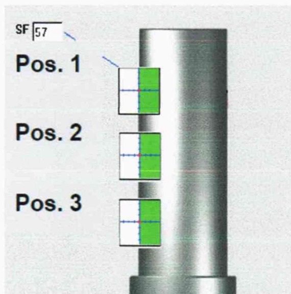
Рисунок 1 – Схема для измерения отклонения от прямолинейности и радиального биения
