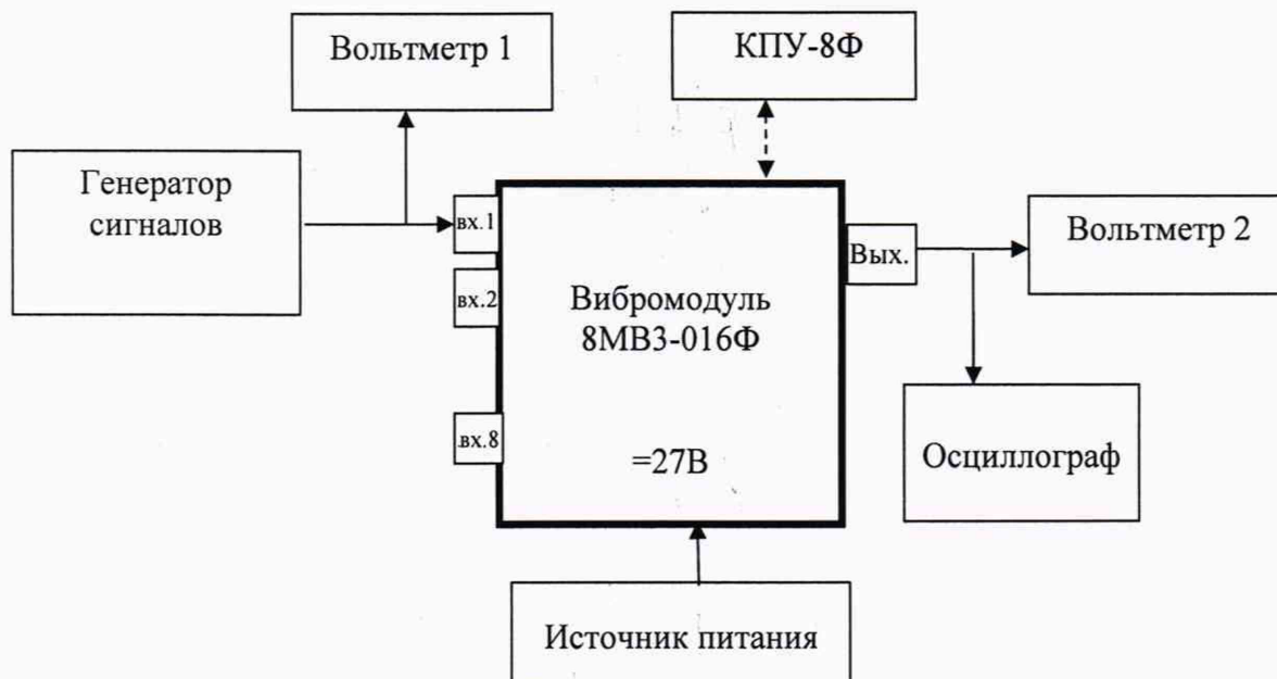
Рисунок 2 - Схема измерения амплитудных и амплитудно-частотных характеристик вибромодуля 8МВ3-016Ф
