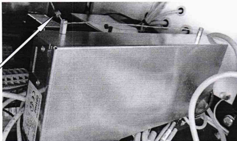
Рисунок 2 - Схема пломбировки от несанкционированного доступа крышки контроллера СРТН02
