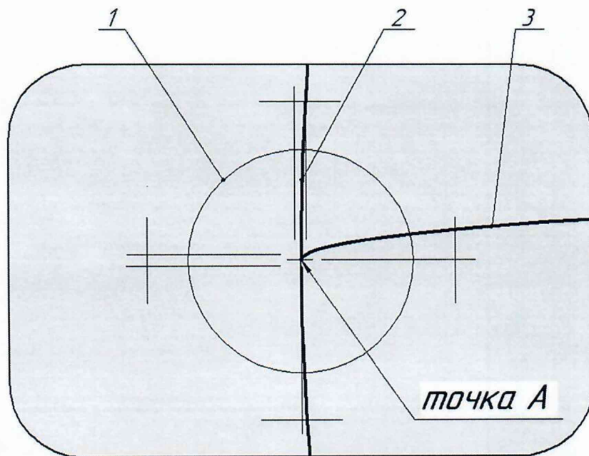
Рисунок А.7 – Схема измерений опорных точек P_0 , P_{ил}
