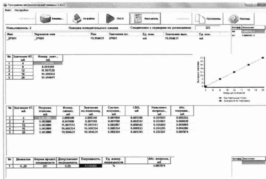
Рисунок 1 - ПО поверки
