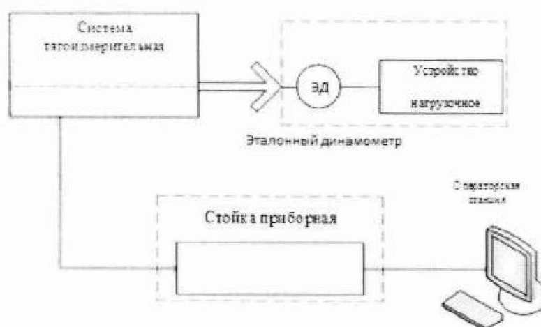
Рисунок 7 – Схема поверки ИК силы от тяги двигателя
