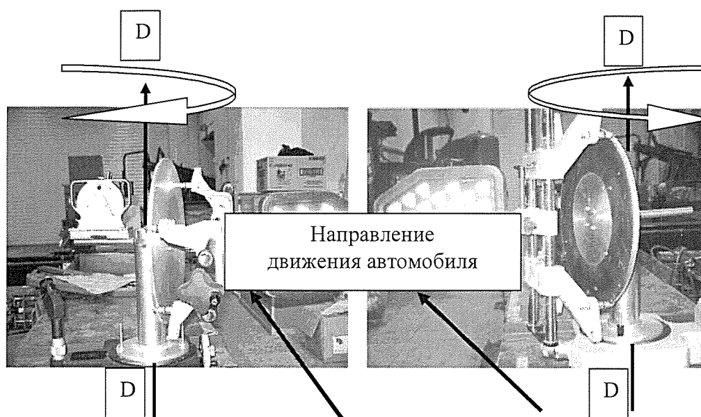
Рисунок 3 - Схема измерений углов индивидуального схождения колес
