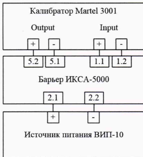
Рисунок 1 - Схема измерений силы постоянного тока
