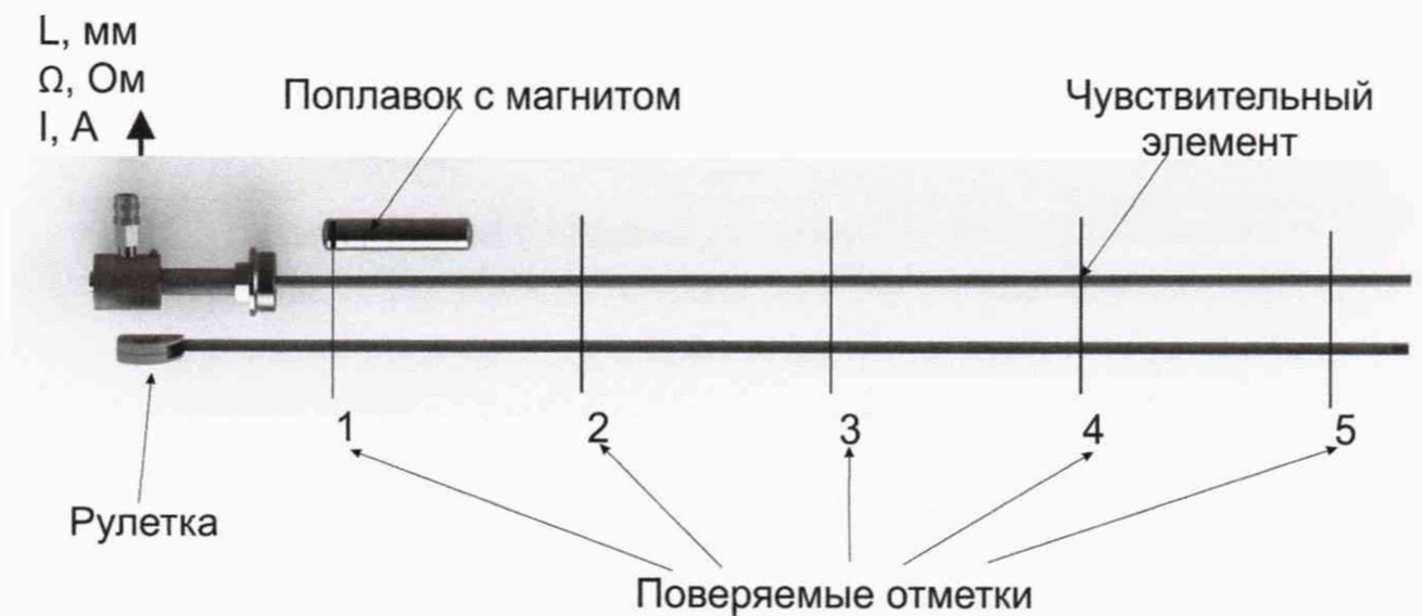
Рисунок 2 – Проверка преобразователя без демонтажа с помощью эталонной рулетки с лотом
