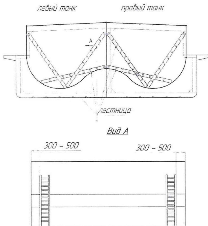
Рисунок А.4 – Схемы расстановки лестниц при измерениях
