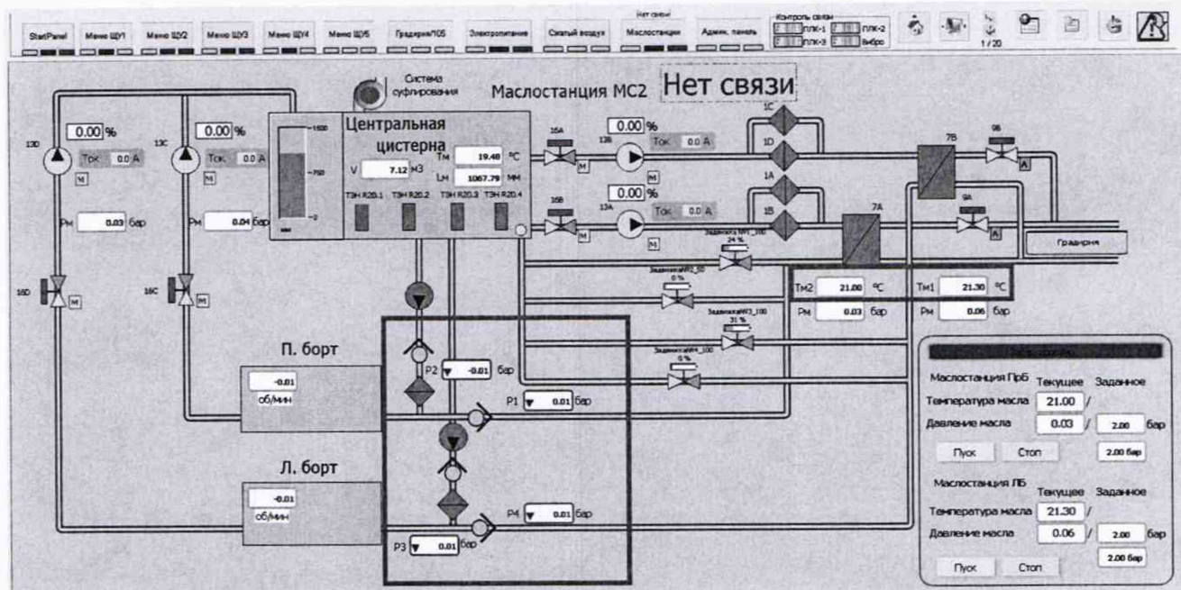
Рисунок 2 Окно с результатами измерений ИК избыточного давления масла на входе в маслоагрегаты или испытываемые изделия
