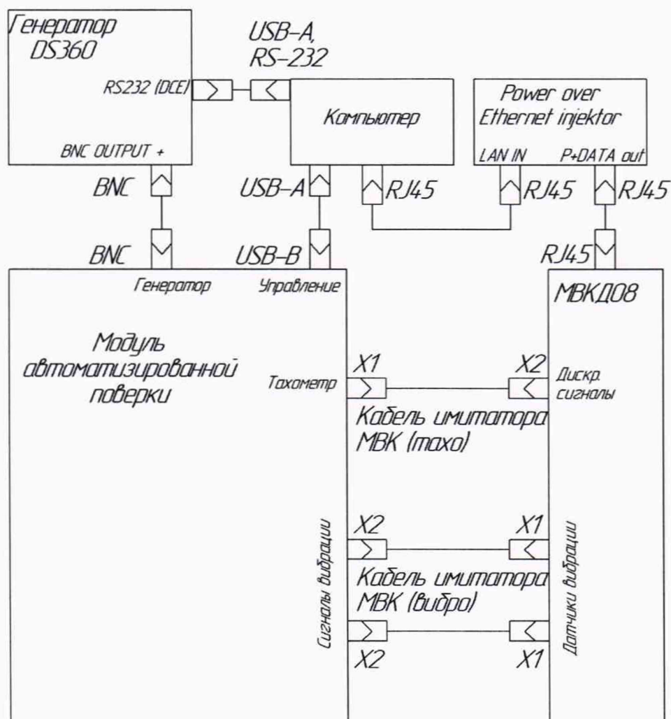
Рисунок 7-2. Схема испытаний.
