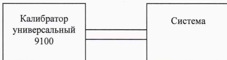
Рисунок 1 – Структурная схема определения погрешностей измерений силы постоянного тока для испытательных сигналов до 20 А
