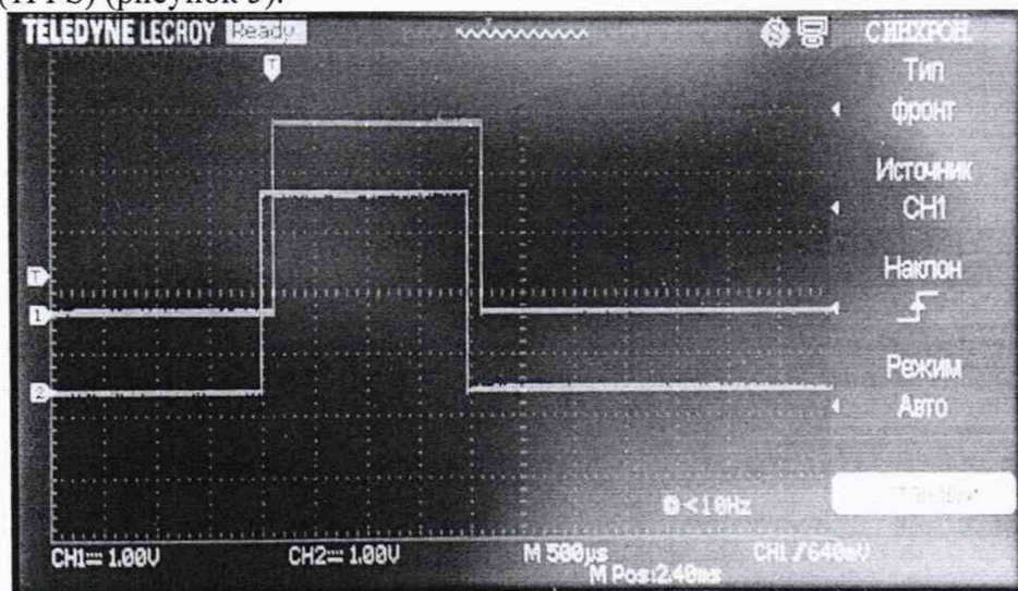
Рисунок 5 - Осциллограмма импульсов 1PPS.
