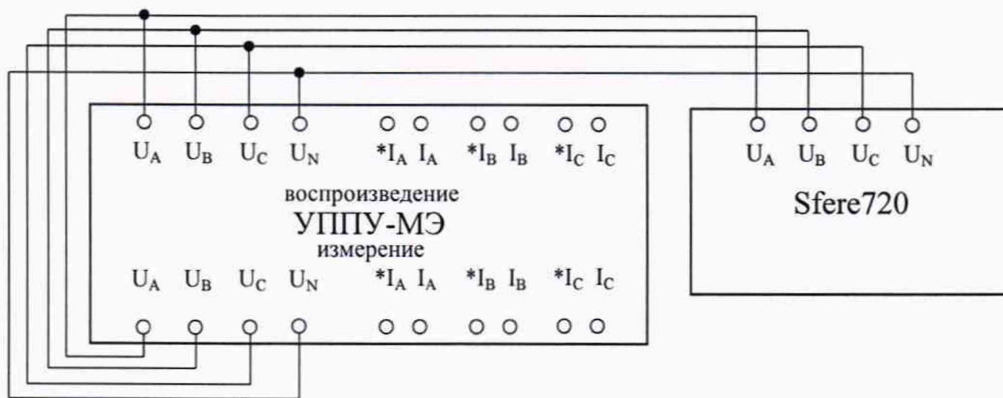
а) Схема подключений при измерении среднеквадратических значений фазного и линейного напряжений переменного тока, частоты переменного тока
