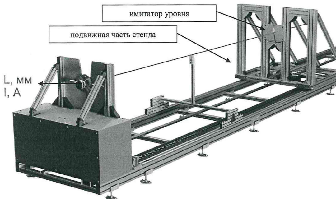
Рисунок 2 - Поверка уровнемера на поверочной установке с имитацией изменения уровня
