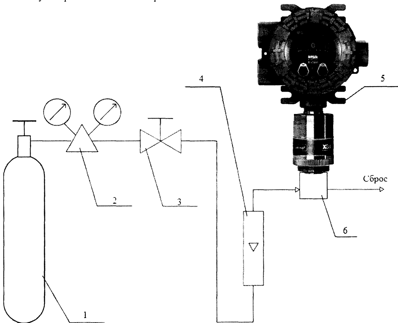
1 – баллон с ГС; 2 – редуктор баллонный; 3 – вентиль точной регулировки трассовой; 4 – ротаметр (индикатор расхода); 5 – газоанализатор; 6 – насадка для подачи ГС
