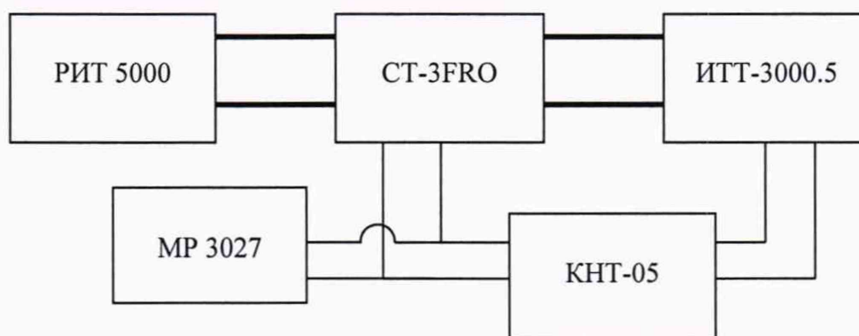
Рисунок 1 – Схема измерений
