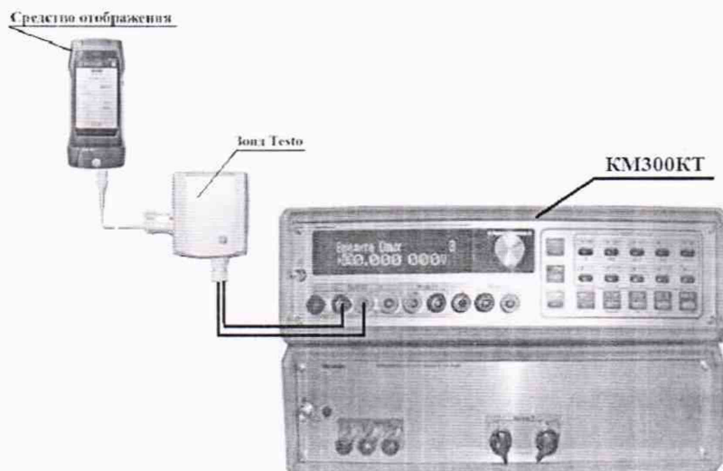
Рисунок 9 – Схема подключения зонда Testo к компаратору-калибратору универсальному KM300KT при определении абсолютной погрешности измерений напряжения постоянного тока
