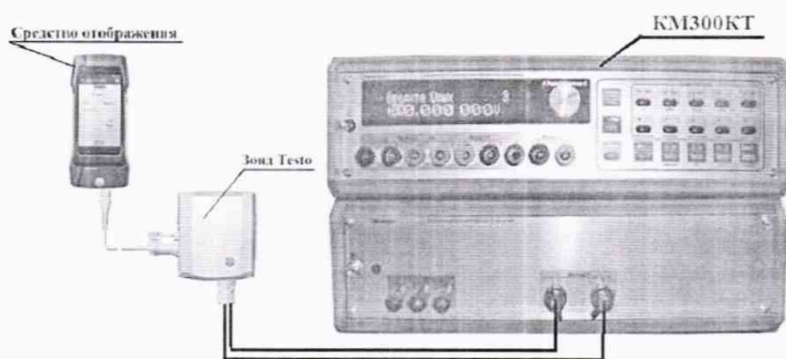
Рисунок 10 – Схема подключения зонда Testo к компаратору-калибратору универсальному KM300KT при определении абсолютной погрешности измерений силы постоянного тока
