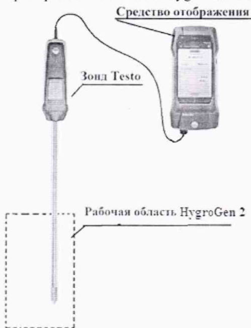
Рисунок 4 – Схема определения абсолютной погрешности измерений относительной влажности методом прямых измерений
