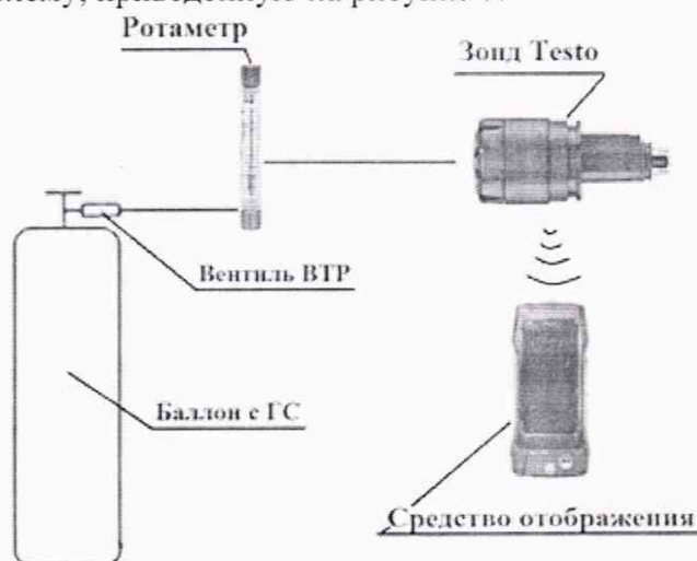
Рисунок 7 – Схема подачи газовых смесей
