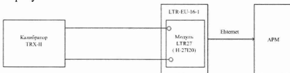
Рисунок 8 – Схема поверки ИК давления для ПП с аналоговым выходом
