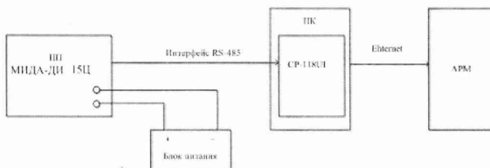
Рисунок 7 – Схема поверки ИК давления для ПП с цифровым выходом
