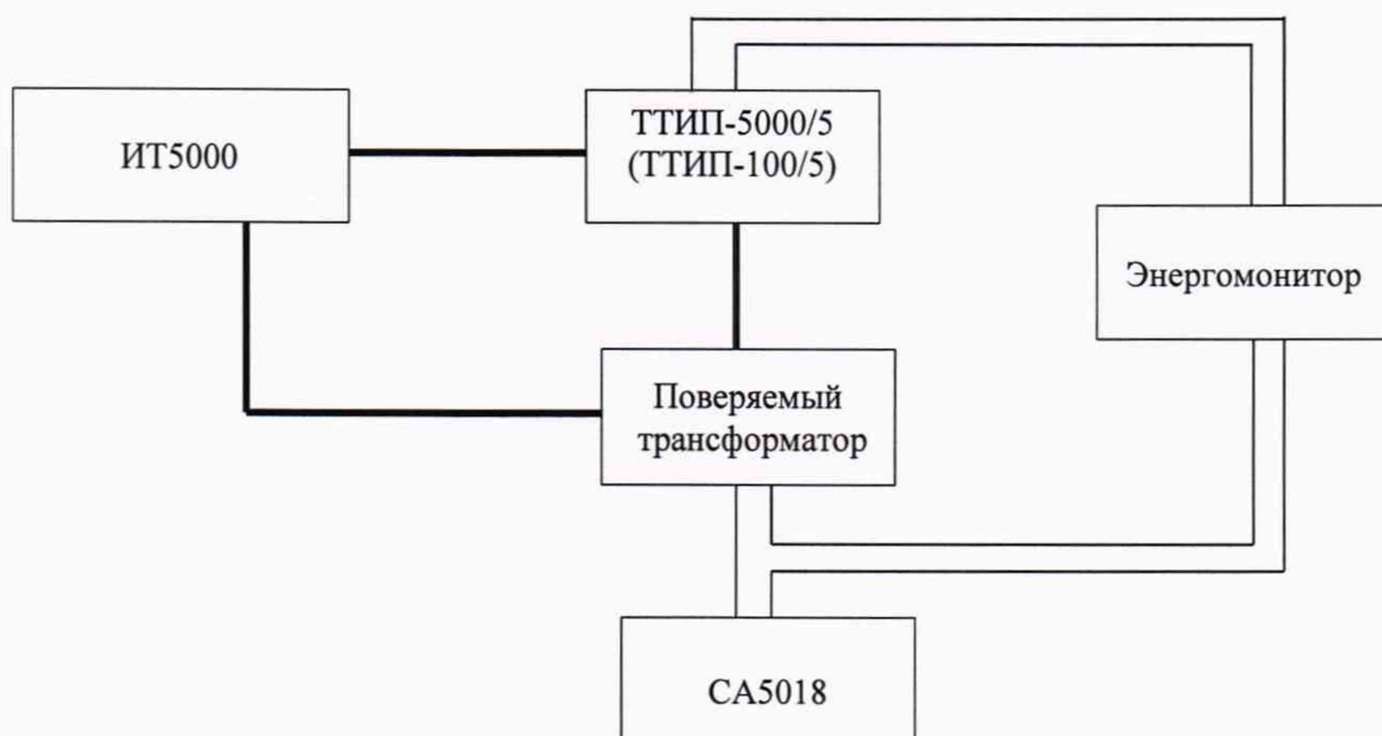
Рисунок 3 – Структурная схема определения погрешностей трансформаторов с номинальным первичным током 120, 3200, 4500 А
