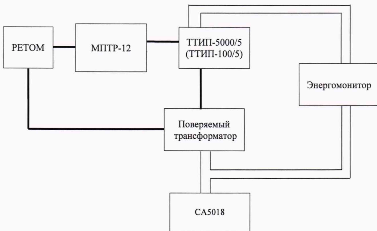
Рисунок 4 – Структурная схема определения погрешностей трансформаторов с номинальным первичным током 5500 А
