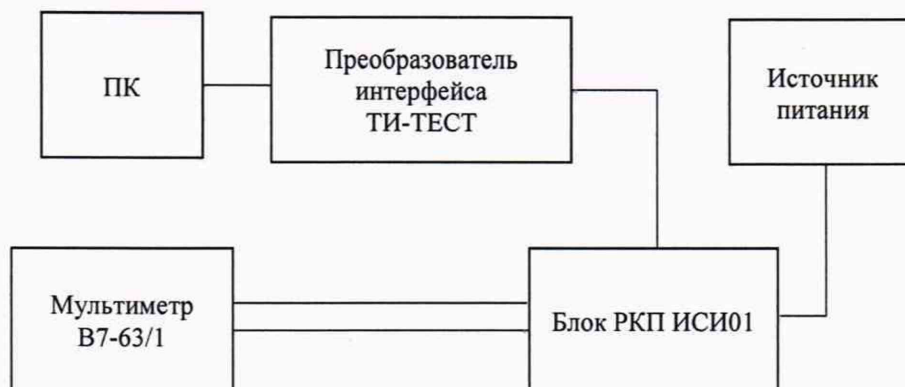
Рисунок 2 - Схема определения абсолютной погрешности воспроизведений напряжения постоянного тока
