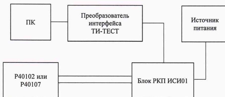
Рисунок 3 - Схема определения относительной основной погрешности измерений электрического сопротивления изоляции
