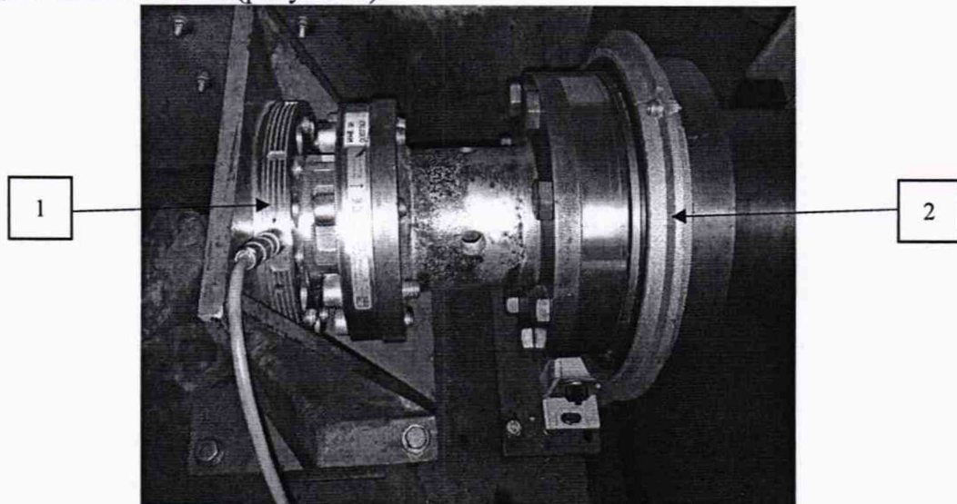
Рисунок 3 – Схема для определения приведенной (к ВП) погрешности измерений крутящего момента силы (1 – датчик крутящего момента ТВ2, 2 – датчик крутящего момента силы T10F)
