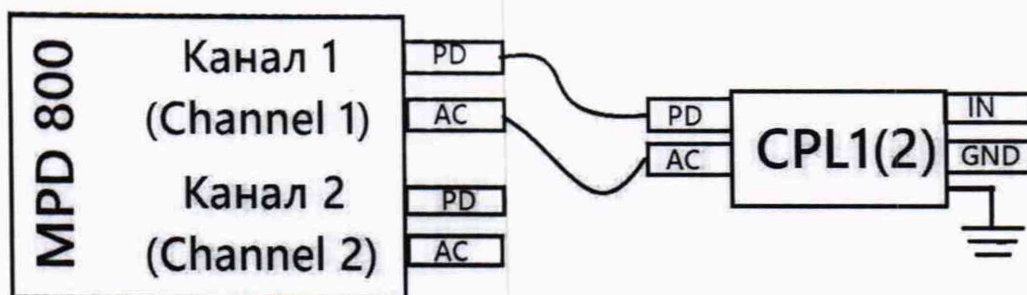
Рисунок 7 – Схема соединения блоков MPD 800 и CPL 1 (CPL 2) при определении относительной погрешности измерений входных среднеквадратических значений силы переменного тока на входе CPL1 (CPL2)
