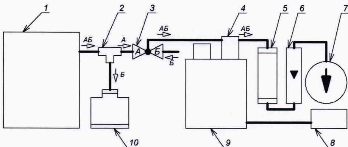
Рисунок 4 – схема установки для поверки газосигнализатора
