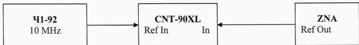
Рисунок 2 – Схема измерения частоты опорного генератора
