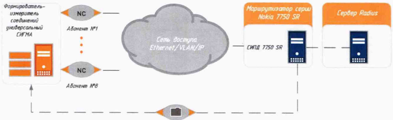
Рисунок 1 – Схема поверки СИПД
