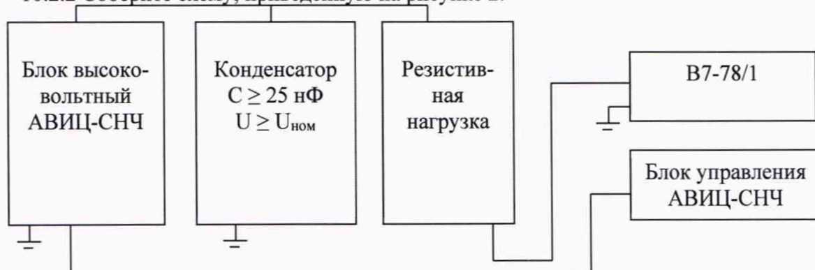
Рисунок 2 – Схема проверки погрешности измерений силы постоянного тока
