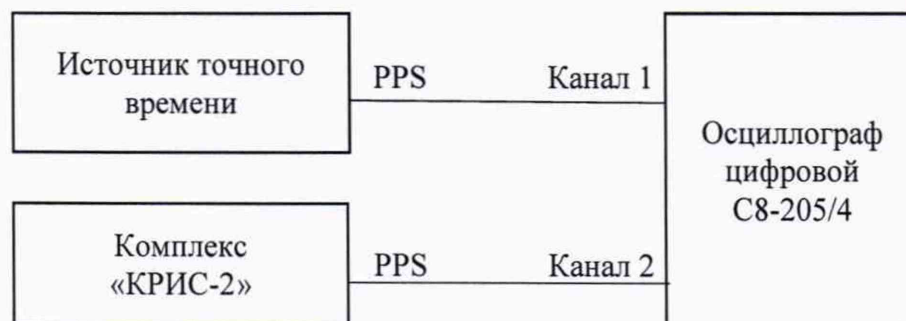
Рисунок 3 – Схема выполнения измерений
