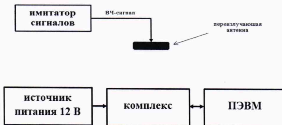
Рисунок 6 - Схема проведения измерений при определении абсолютной инструментальной погрешности определения координат
