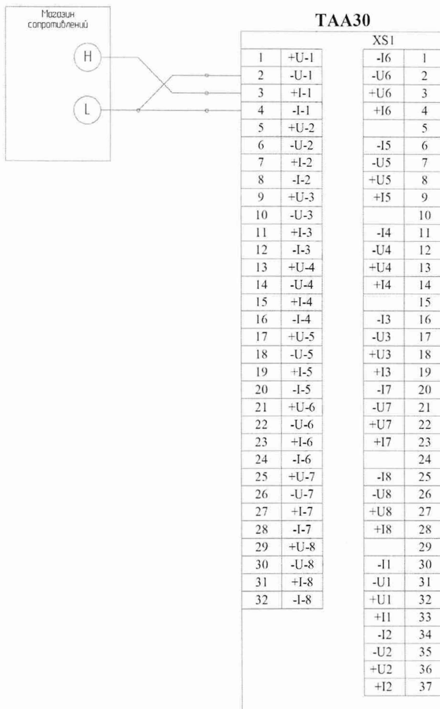
Рисунок А.7 – Пример подключения имитатора (магазин сопротивлений) к модулю АИ102 через полевой адаптер ТAA30 для задания сигналов имитации термопреобразователей ТСМ и ТСП, подключенных по трехпроводной схеме подключения
