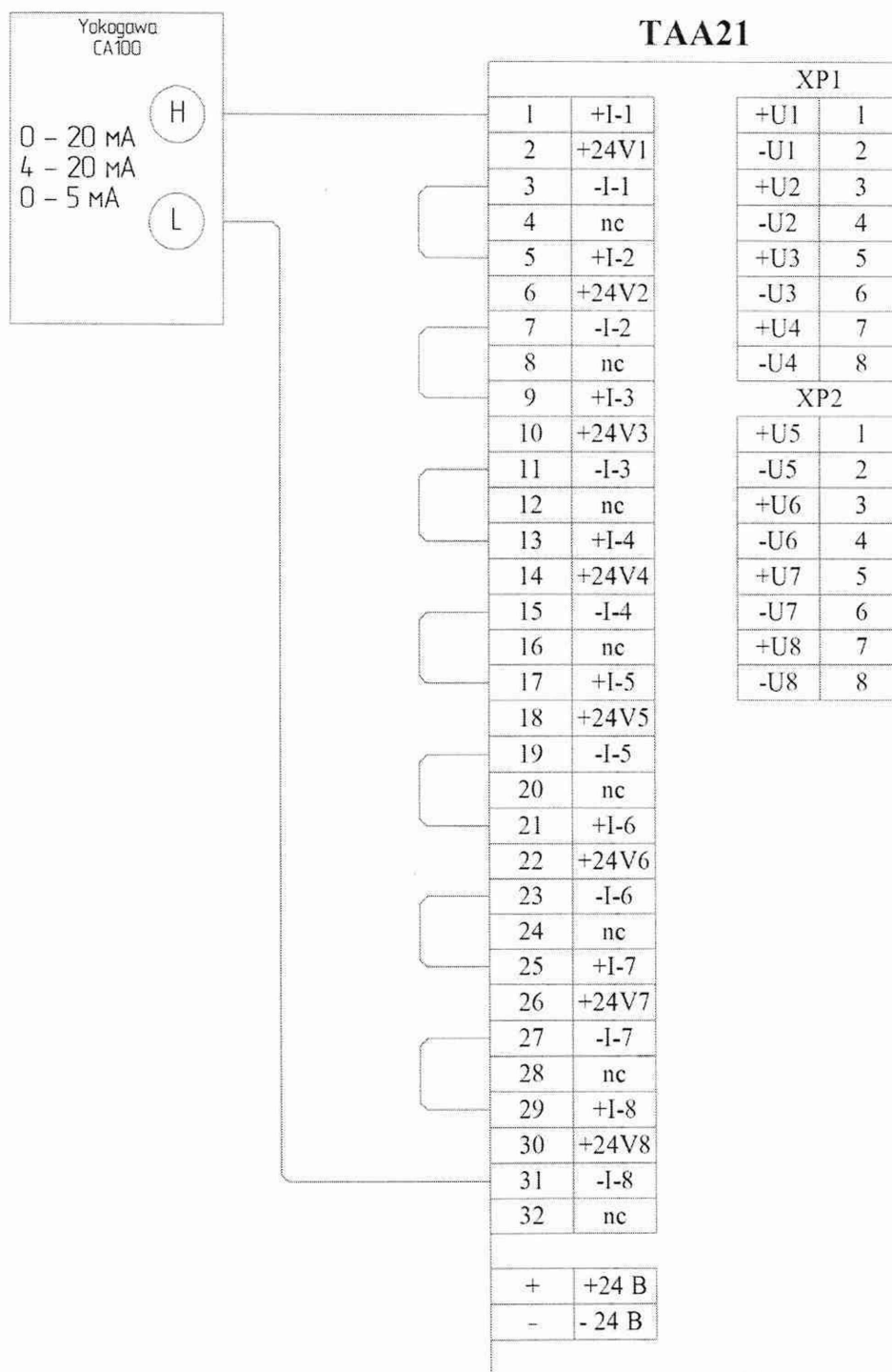
Рисунок А.2 – Пример подключения имитатора (Yokogawa CA100) к модулю AI101 через полевой адаптер ТАА21 для задания сигналов имитации токовых датчиков (4-20) мА, (0-20) мА или (0-5) мА с автономным питанием
