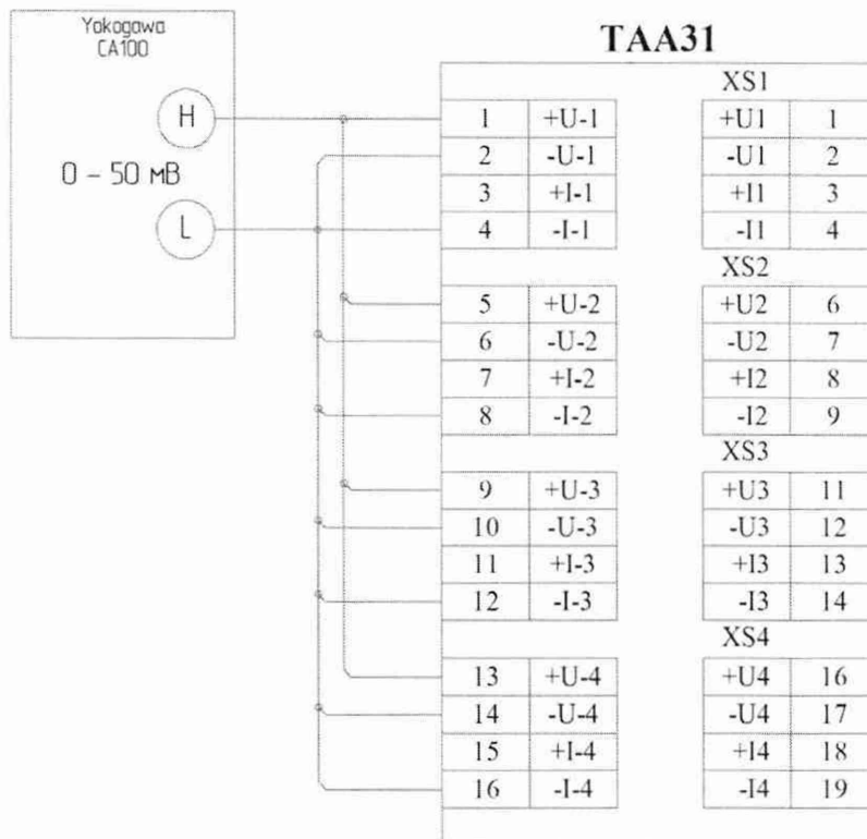
Рисунок А.10 – Пример подключения имитатора (Yokogawa CA100) к модулю АП104 через полевой адаптер ТAA31 для задания сигналов имитации напряжения постоянного тока (0-50) мВ
