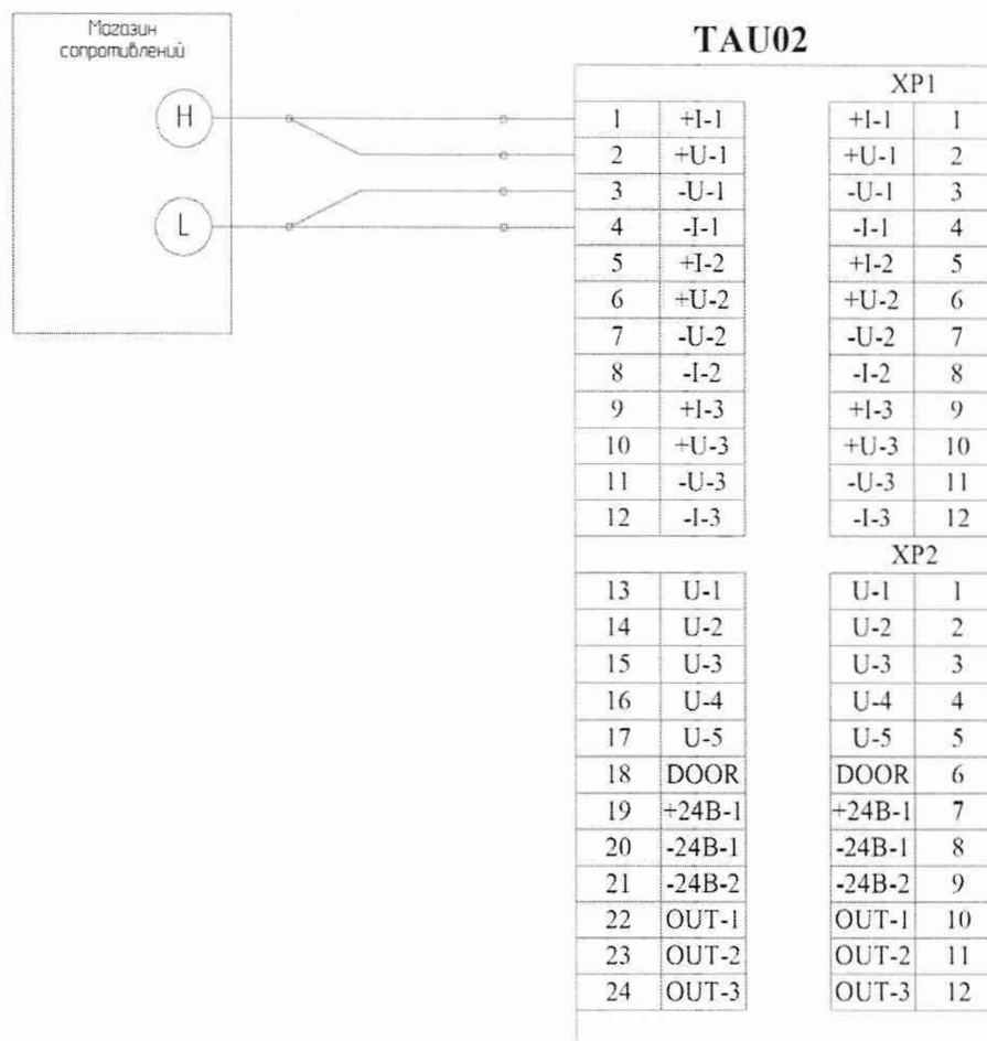
Рисунок А.13 – Пример подключения имитатора (магазин сопротивлений) к модулю SM101 через полевой адаптер ТАУ02 для задания сигналов имитации температуры холодного спая (термопреобразователи сопротивления по ГОСТ6651-2009: Pt-100 \alpha=0,00385 с четырехпроводной схемой подключения)
