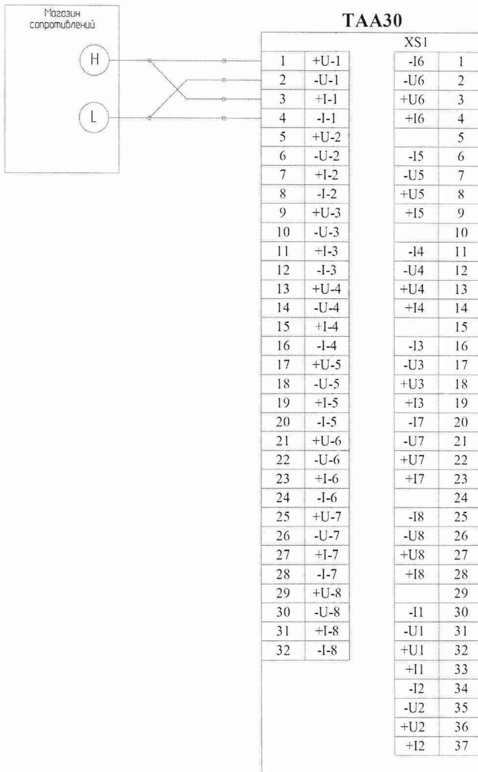
Рисунок А.8 – Пример подключения имитатора (магазин сопротивлений) к модулю АИ102 через полевой адаптер ТАА30 для задания сигналов имитации термопреобразователей ТСМ и ТСР, подключенных по четырехпроводной схеме подключения
