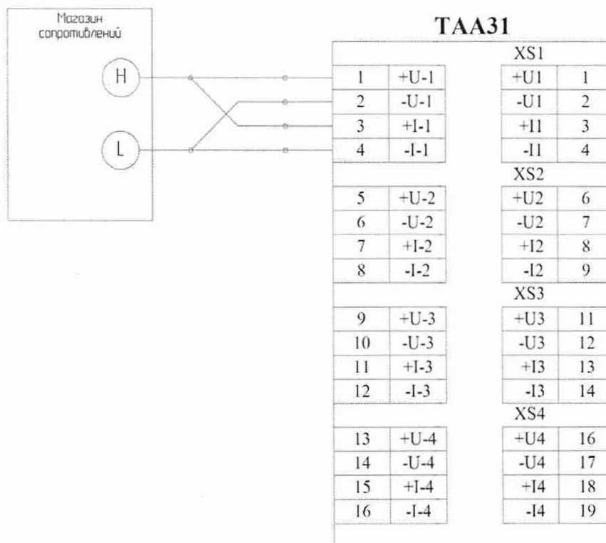
Рисунок А.12 – Пример подключения имитатора (магазин сопротивлений) к модулю АИ104 через полевой адаптер ТAA31 для задания сигналов имитации термопреобразователей ТСМ и ТСП, подключенных по четырехпроводной схеме подключения
