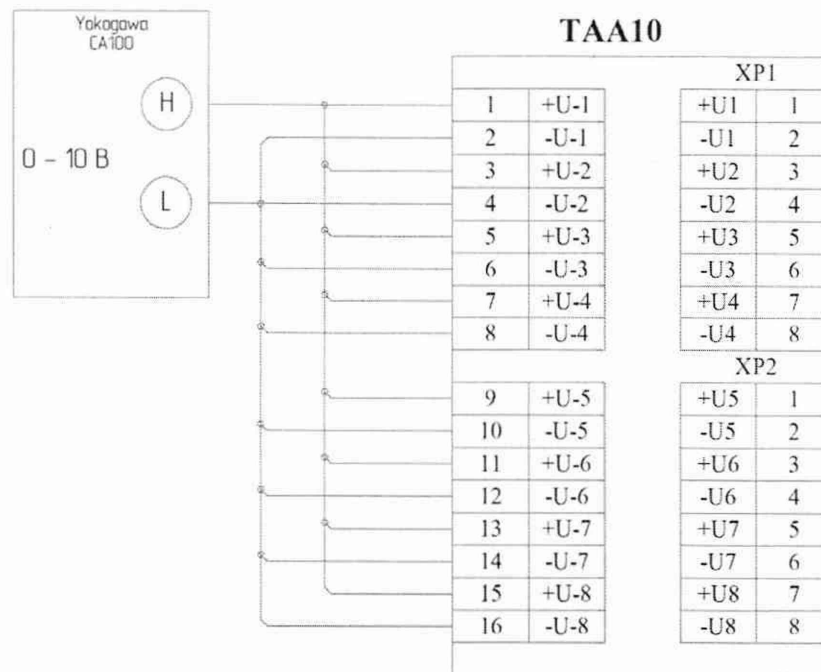
Рисунок А.4 – Пример подключения имитатора (Yokogawa CA100) к модулю АИ101 через полевой адаптер ТАА10 для задания сигналов имитации датчиков напряжения (0-10) В
