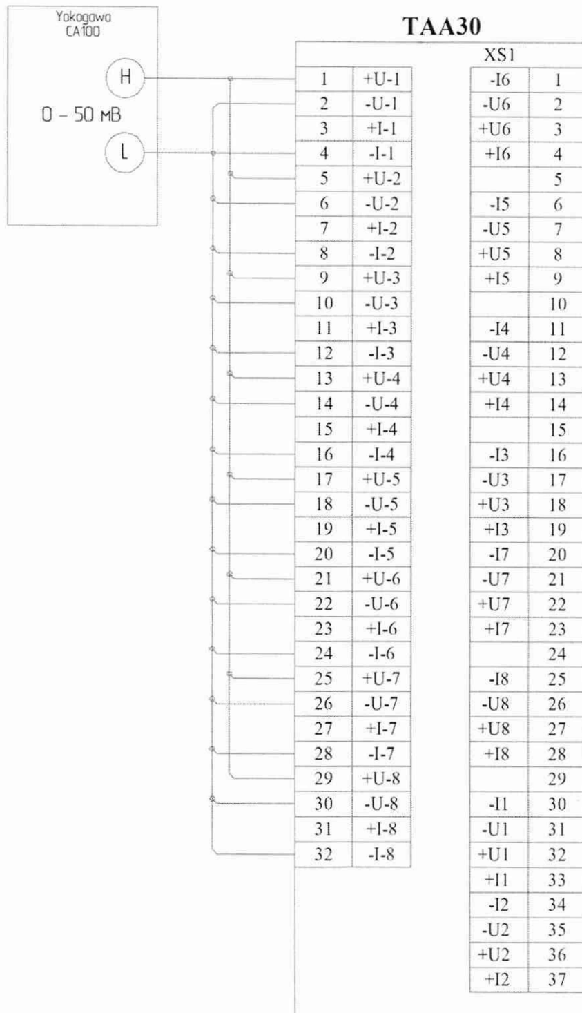
Рисунок А.5 – Пример подключения имитатора (Yokogawa CA100) к модулю AI102 через полевой адаптер ТАА30 для задания сигналов имитации ЭДС термопар ТХА, ТХК, ТПР (тип В), ТПП (тип S), ТПП (тип R)
