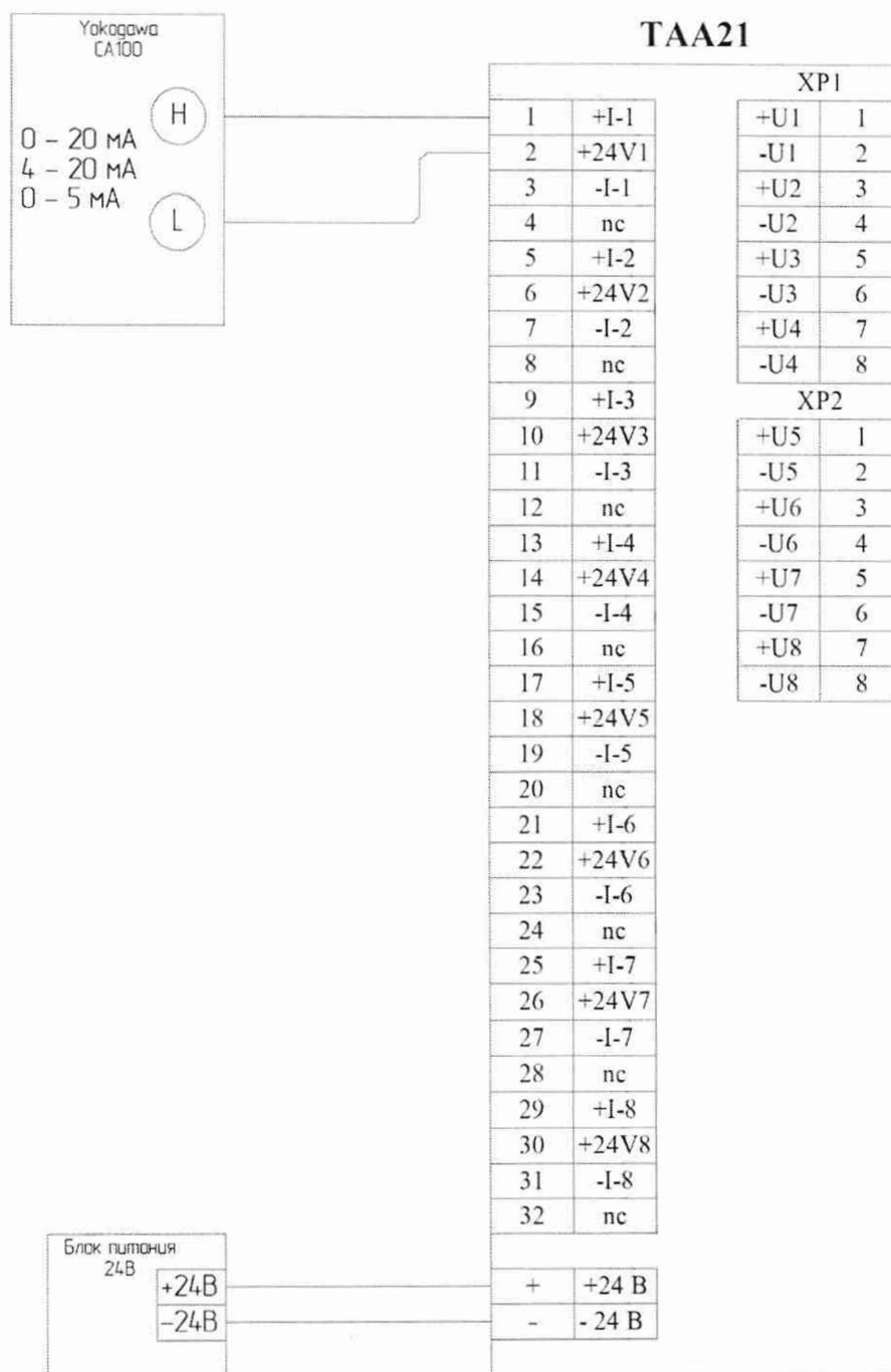
Рисунок А.1 – Пример подключения имитатора (Yokogawa CA100) к модулю АИ101 через полевой адаптер ТАА21 для задания сигналов имитации токовых датчиков (4-20) мА, (0-20) мА или (0-5) мА с питанием от контроллера Elicont-100
