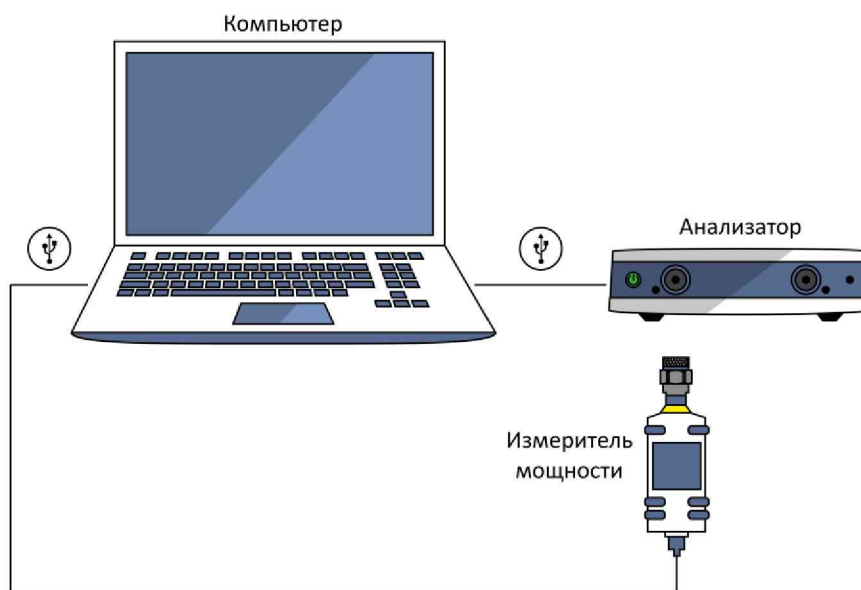
Рисунок А.4 – Схема измерений
