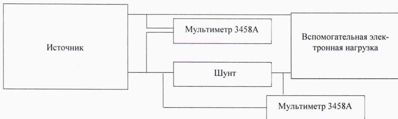
Рисунок 4 - Структурная схема определения нестабильности выходного напряжения постоянного тока, вызванной изменением силы тока в нагрузке, и нестабильности силы выходного тока, вызванной изменением напряжения на нагрузке (от 0 до 1000 В включ.)
