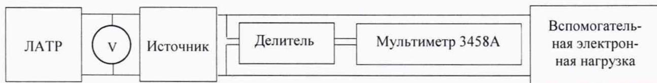
Рисунок 6 - Структурная схема определения нестабильности выходного напряжения постоянного тока, вызванной изменением напряжения питания (от 0 до 1000 В включ.)
