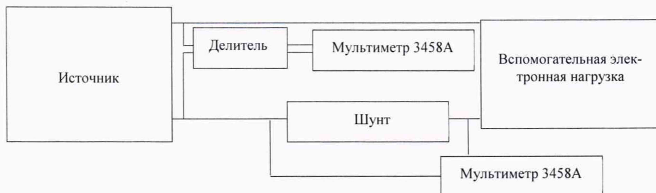
Рисунок 5 - Структурная схема определения нестабильности выходного напряжения постоянного, вызванной изменением силы тока в нагрузке, и нестабильности силы выходного тока, вызванной изменением напряжения на нагрузке (св. 1000 В)
