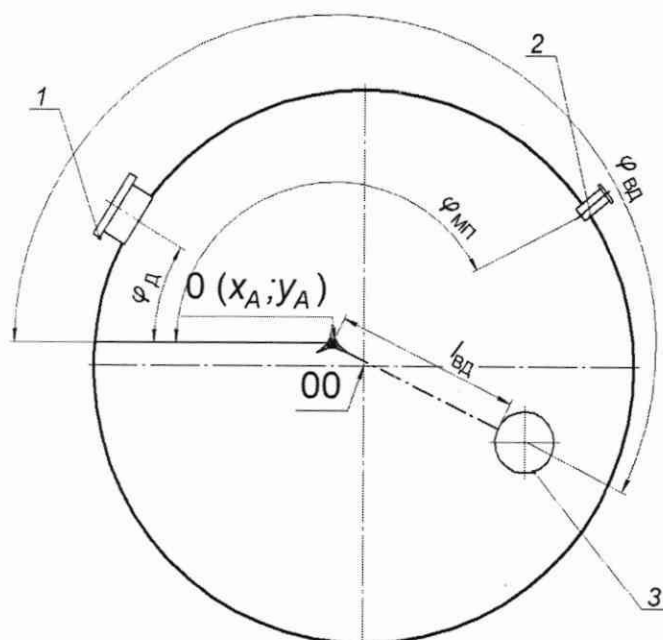
1 – люк-лаз; 2 – приемо-раздаточный патрубок, 3 – внутренняя деталь цилиндрической формы; $00$ – центр днища резервуара; $0(x_A; y_A)$ – точка установки станции
