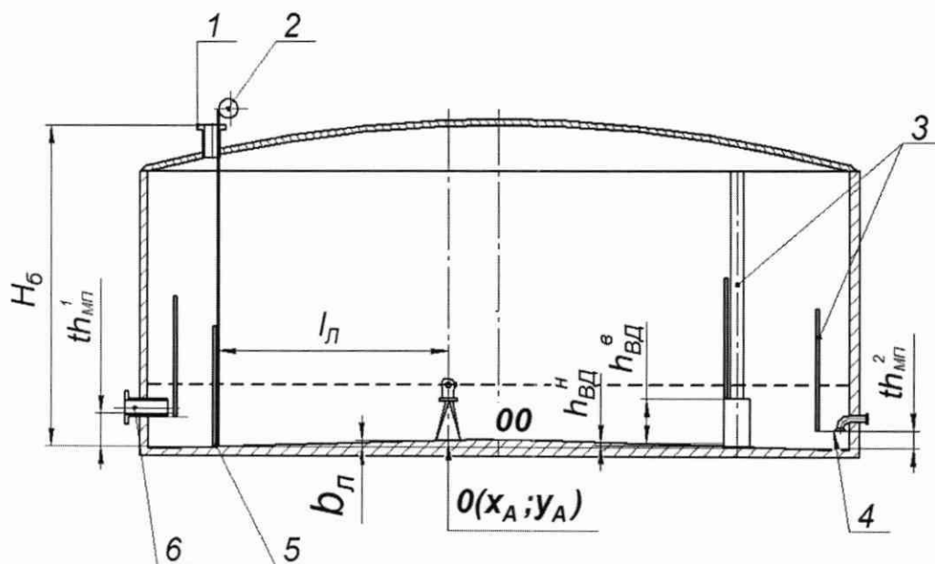
1 – измерительный люк; 2 – измерительная рулетка с грузом; 3 – точки установки рейки; 4 – ПРУ; 5 – точка касания днища грузом рулетки; 6 – ПРП
