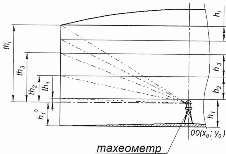
Рисунок А.5 – Схема образующих резервуара
