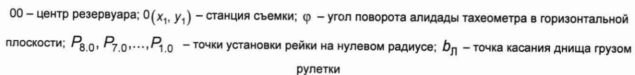
Рисунок А.7 – Координаты отсчета (место установки вехи) неровностей днища и точки касания днища грузом рулетки
