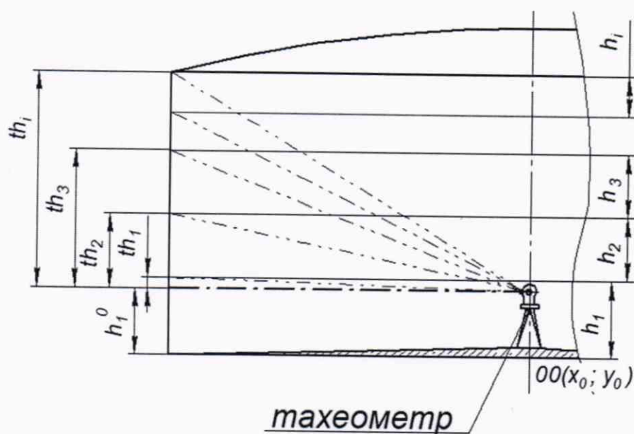
Рисунок А.5 – Схема образующих резервуара
