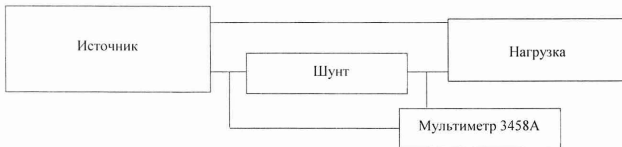
Рисунок 2 – Структурная схема определения абсолютной погрешности измерений/установки силы постоянного тока
