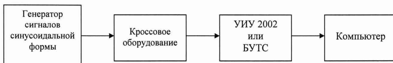
Рисунок 7 - Схема определения метрологических характеристик ИК частоты переменного тока и ИК частоты переменного тока, соответствующей значениям частоты вращения роторов
