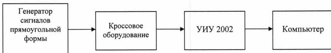
Рисунок 15 - Схема определения метрологических характеристик ИК интервала времени
