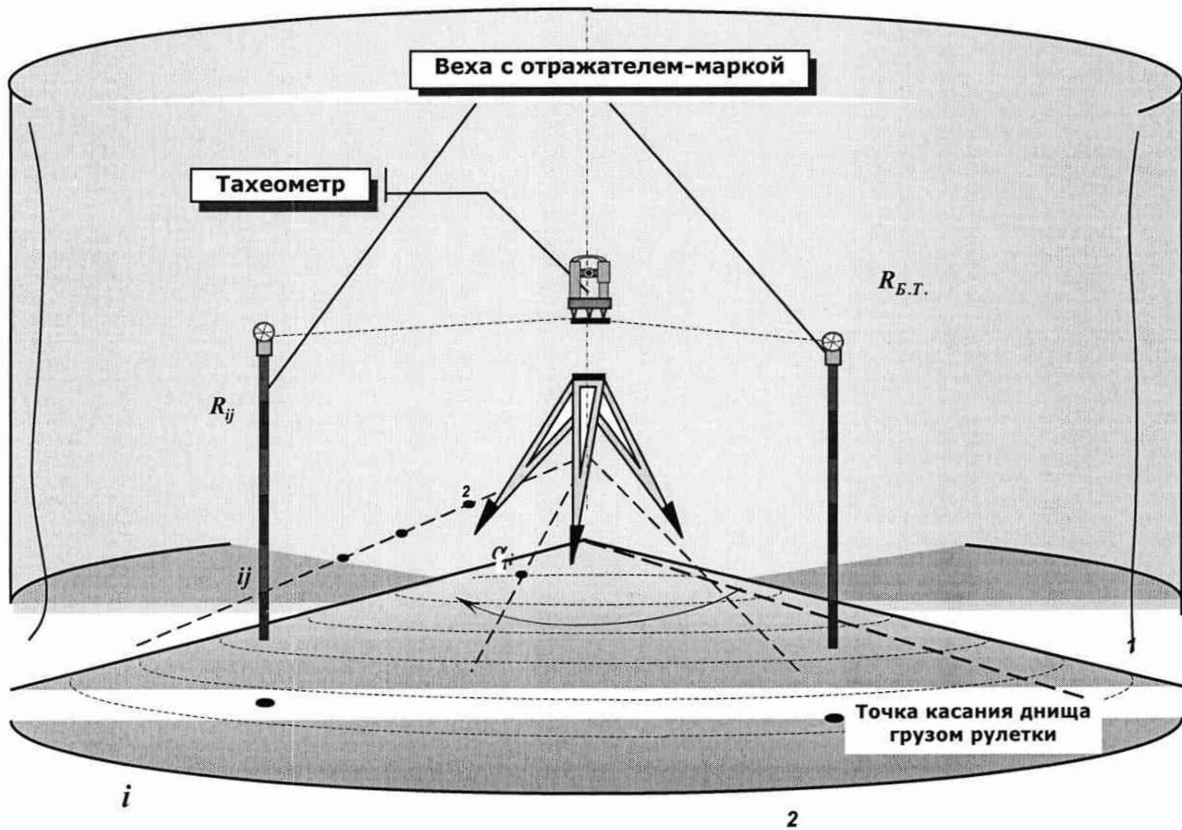
Рисунок А.6 Измерения при определении параметров днища резервуара
