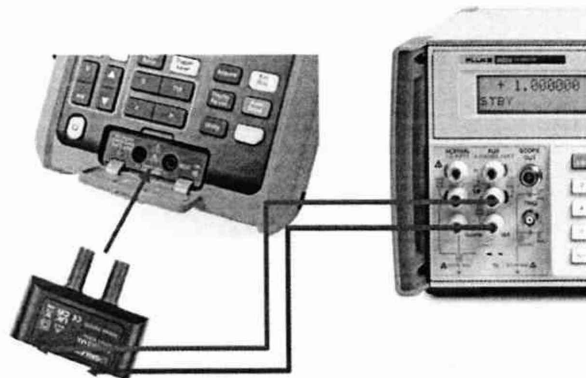
Токовый шунт 10 А
