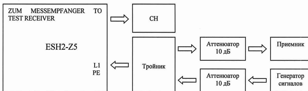
Рисунок 1. Схема калибровки выходного уровня генератора сигналов
