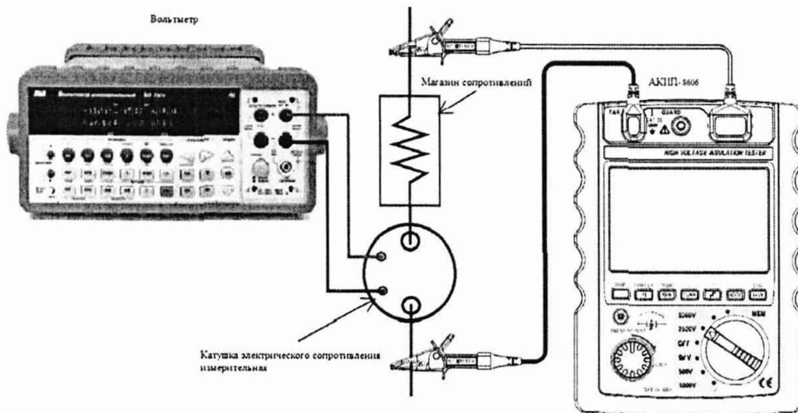
Рисунок 1 – Схема подключения измерителя сопротивления при поверке
