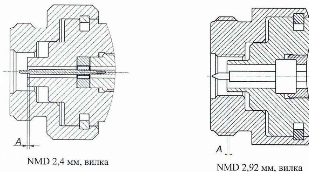
Рисунок А.2 – Присоединительный размер А
