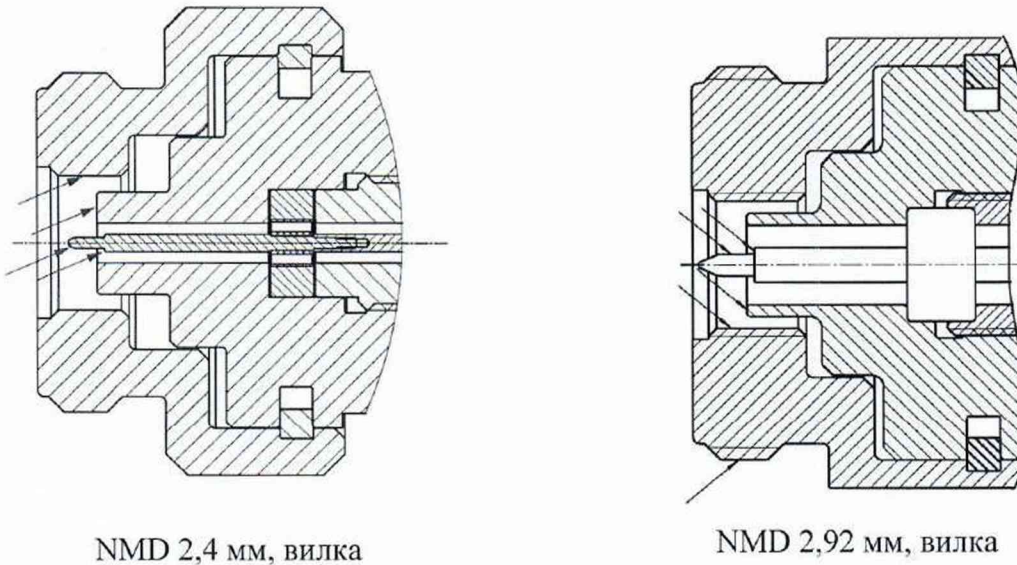
Рисунок А.1 – Чистка соединителей
