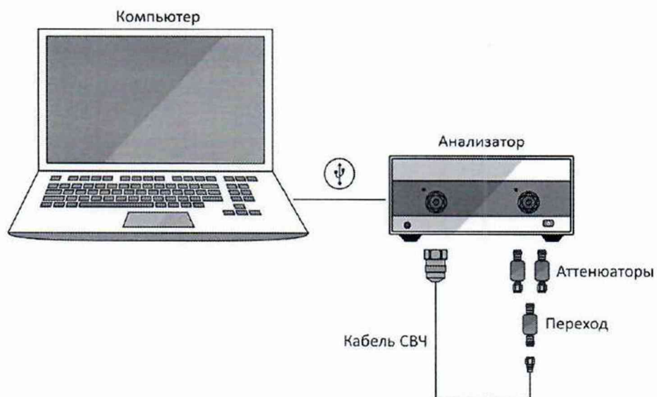
Рисунок А.11 – Схема измерений
