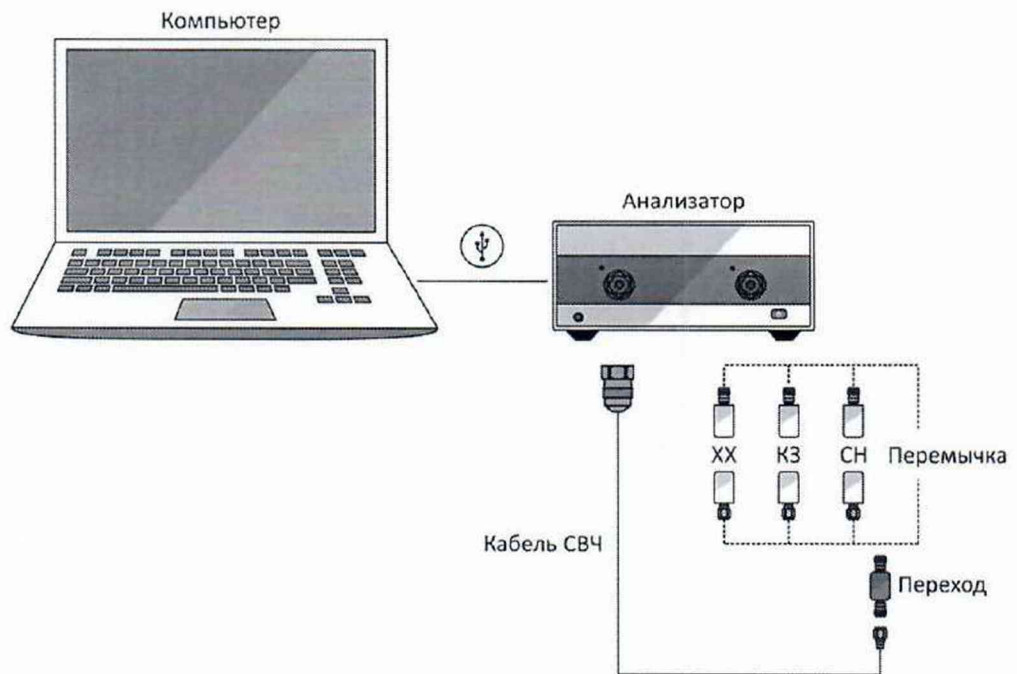
Рисунок А.10 – Схема измерений (проведение «калибровки»)
