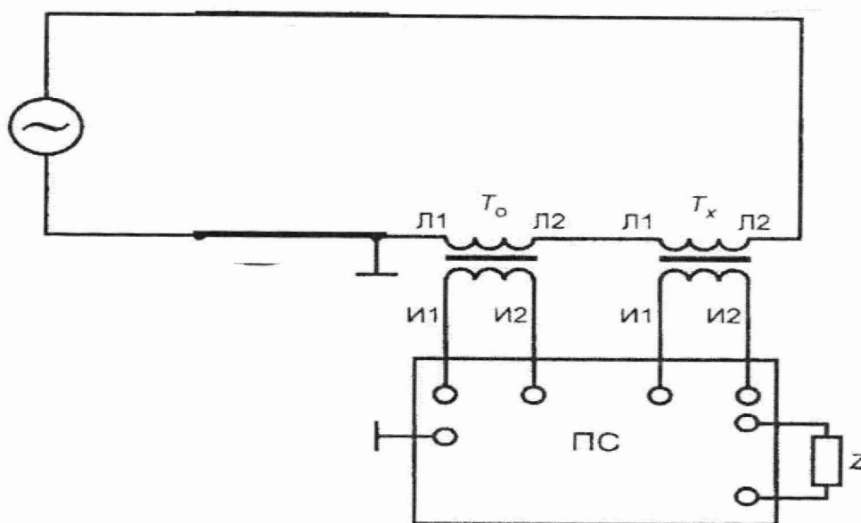
Рисунок 1 Схема поверки с использованием рабочего эталона и прибора сравнения ~ – генератор; T_0 — рабочий эталон; T_x — поверяемый трансформатор тока; L_1, L_2 — контактные зажимы первичной обмотки; I_1, I_2 — контактные зажимы вторичной обмотки; Z — нагрузка; ПС — прибор сравнения
