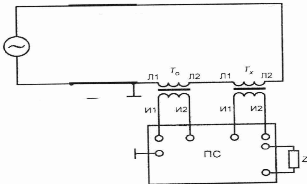
Рисунок 1 Схема проверки с использованием рабочего эталона и прибора сравнения ~ – генератор; T_0 — рабочий эталон; T_x — поверяемый трансформатор тока; L_1, L_2 — контактные зажимы первичной обмотки; I_1, I_2 — контактные зажимы вторичной обмотки; Z — нагрузка; ПС — прибор сравнения
