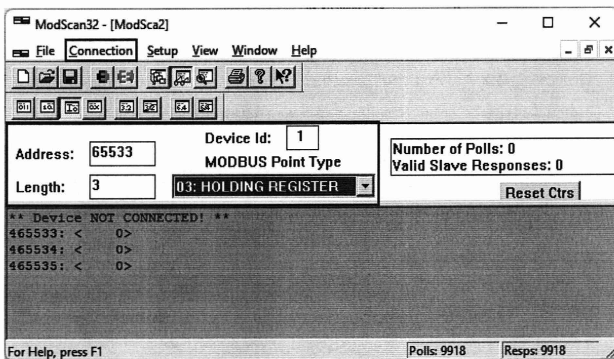
Рисунок 4 – Окно программы для просмотра регистров памяти
