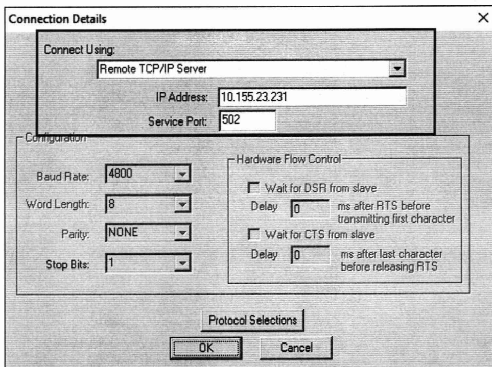
Рисунок 5 – Окно настроек соединения с контроллером
