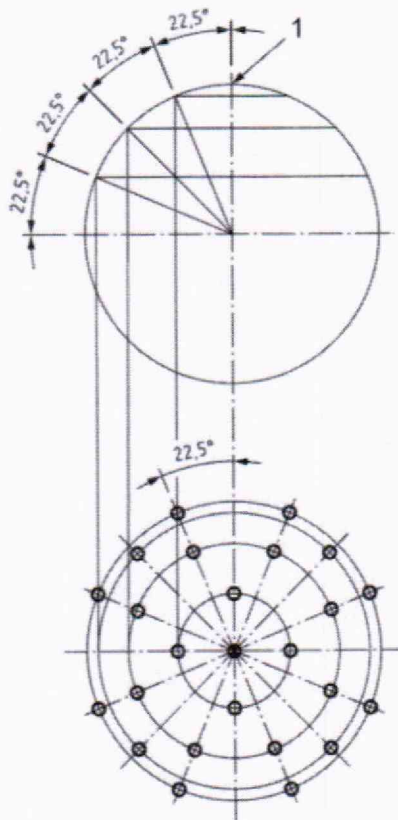
Рисунок 1 – Точки касания на сфере для определения абсолютной погрешности измерительной головки, МРЕР
